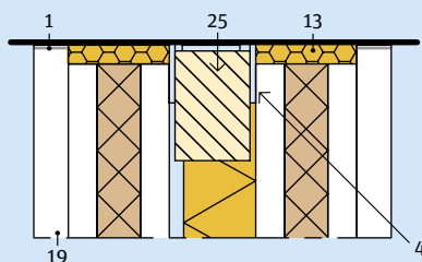
4.13.2 Plafondaansluiting
