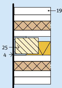
4.13.5 Wandaansluiting
