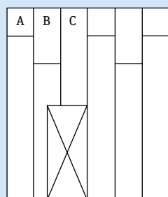
2.9.7 VP70 hoogteoplossing (andere wandtypen in overleg met Faay Vianen)
