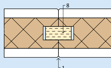
2.6.2 Koppeling
