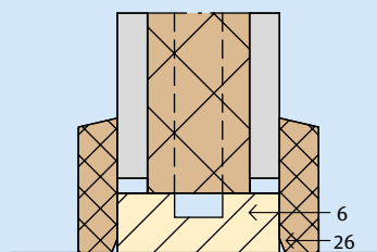
2.14.6 Vloeraansluiting
