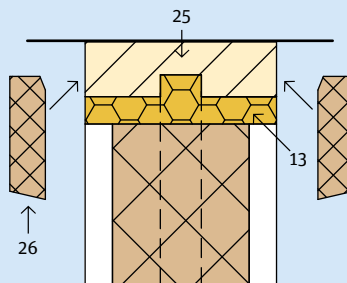
2.9.2 Plafondaansluiting
