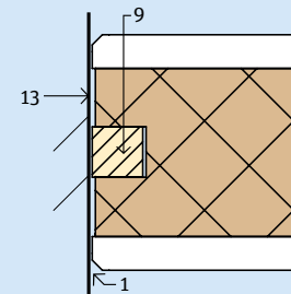
2.8.3 Wandaansluiting
