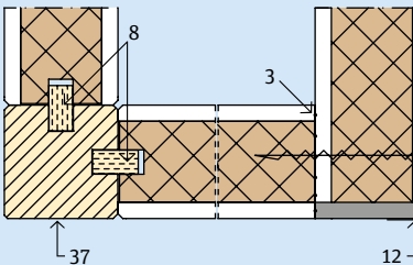
2.8.4 Hoekverbinding
