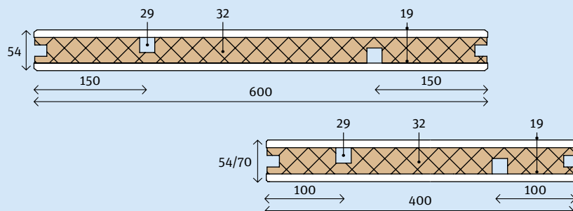
2.6.1 Opbouw wandelement
