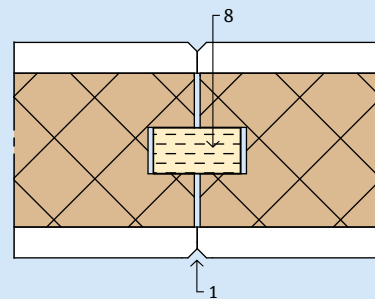
2.8.2 Koppeling
