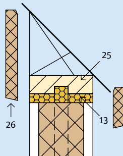
2.9.4 Plafondaansluiting
