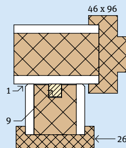
2.8.6 Ontmoeting / kozijnaansluiting / beëindiging
