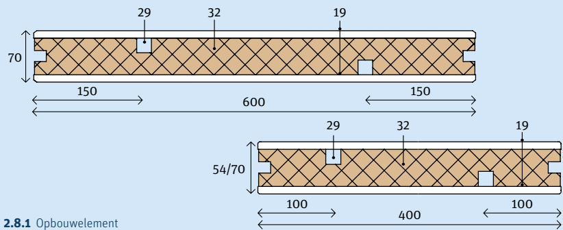
2.8.1 Opbouwelement
