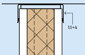
2.7.5 Plafondaansluiting
