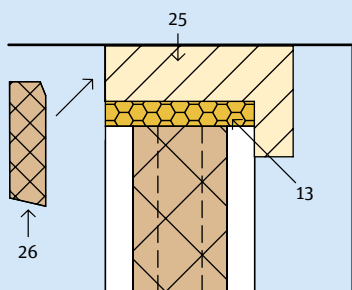
2.7.3 Plafondaansluiting
