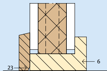
2.7.6 Vloeraansluiting
