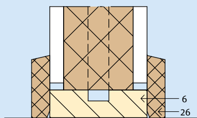
2.9.5 Vloeraansluiting
