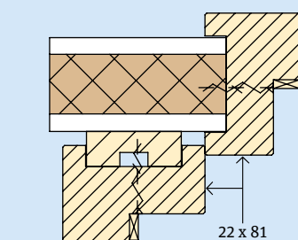
2.6.6 Kozijnaansluiting
