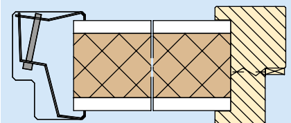
2.8.5 Kozijnaansluiting
