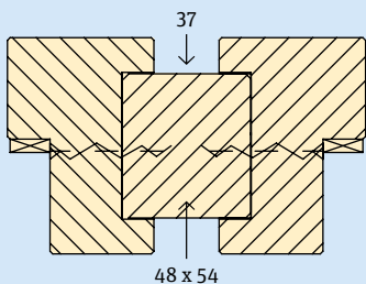
2.7.1 Tussenstijl
