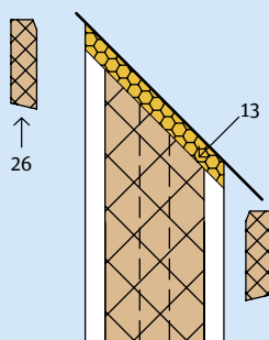
2.9.3 Plafondaansluiting
