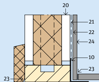
2.7.8 Vloeraansluiting natte cel
