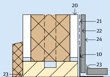
2.9.6 Vloeraansluiting natte cel
