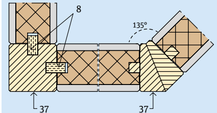
2.14.3 Hoekverbinding
