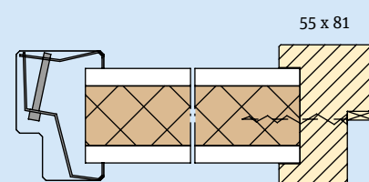
2.6.5 Kozijnaansluiting
