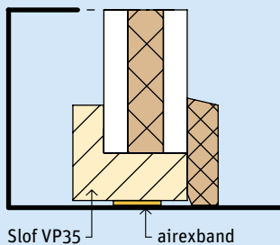
3.9.2 Vloeraansluiting
