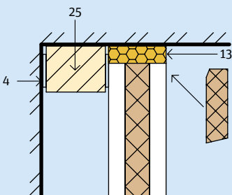
3.9.6 Plafondaansluiting
