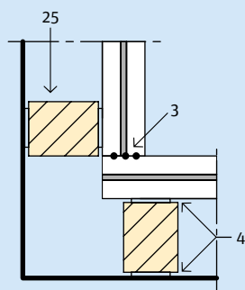
3.7.3 Wandaansluiting/Hoek
