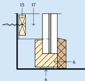
3.7.5 Vloeraansluiting
