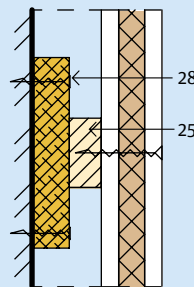
3.9.5 Hoekaansluiting
