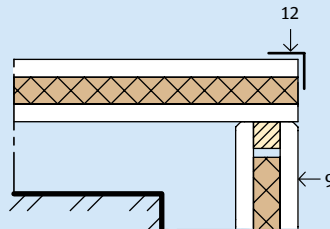
3.9.5 Hoekaansluiting
