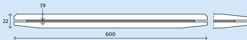
3.7.1 Opbouw wandelement
