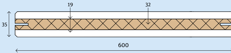
3.9.1 Doorsnede VP35
