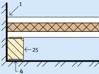
3.9.4 Wandaansluiting
