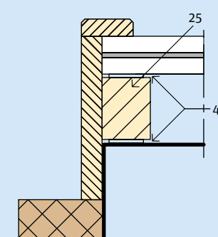
3.7.4 Kozijnaansluiting
